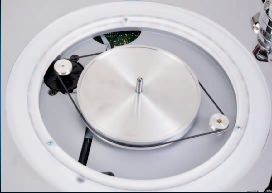
INNERE SCHÖNHEIT: Der Teller rotiert auf einem Lager aus Bronze, der Riemen wird über einen zweiten, passiven Außen-Pulley gespannt.
