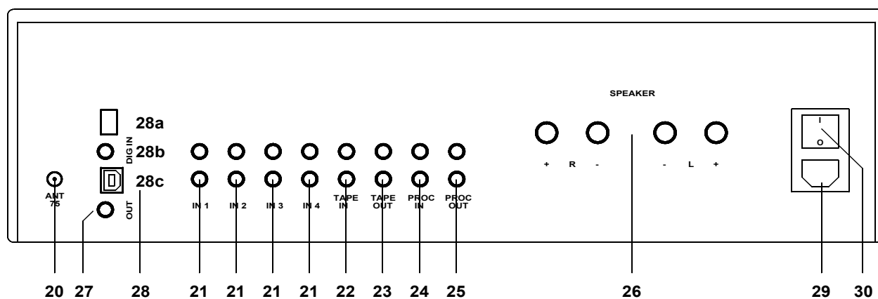
Rückwand
