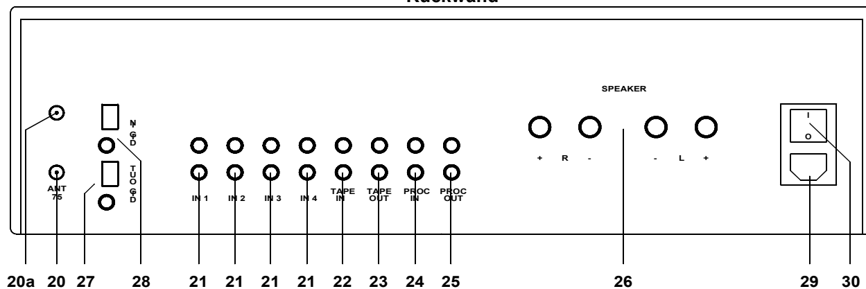
Rückwand
